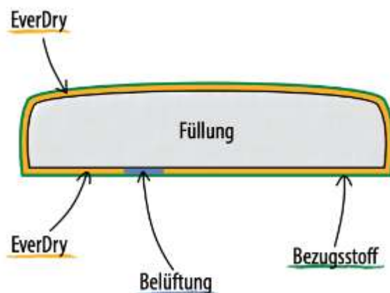
Abbildung: Aufbau Kissen mit EverDry-System
